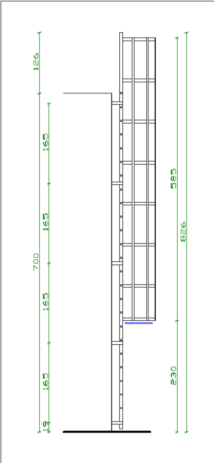
Bočni presjek:
