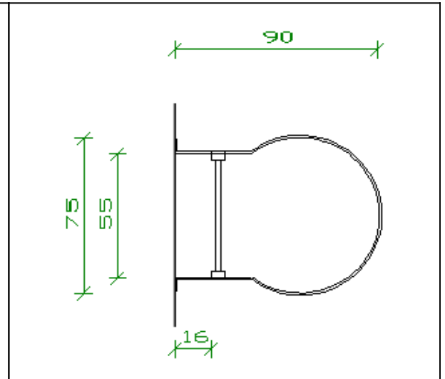
Tlocrt:
