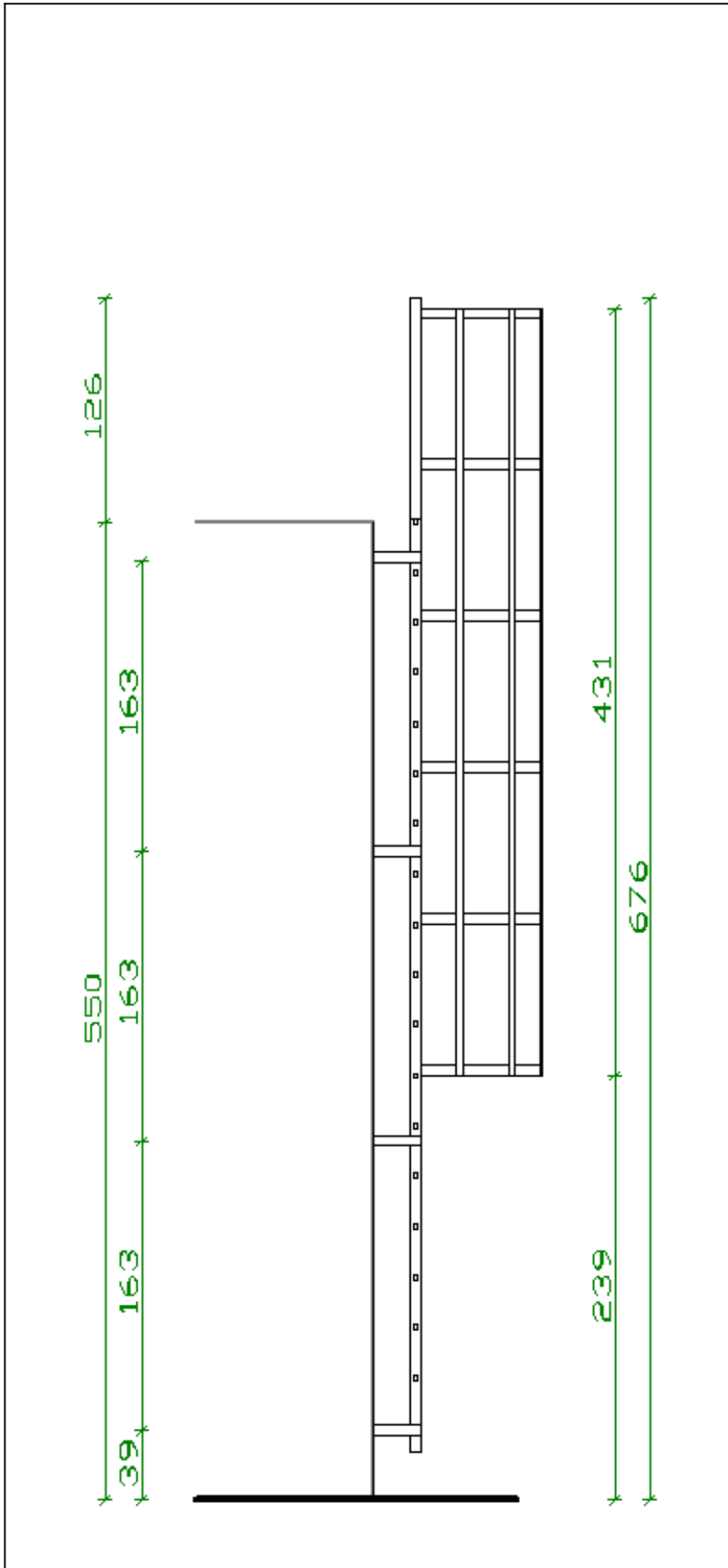
Bočni presjek:
